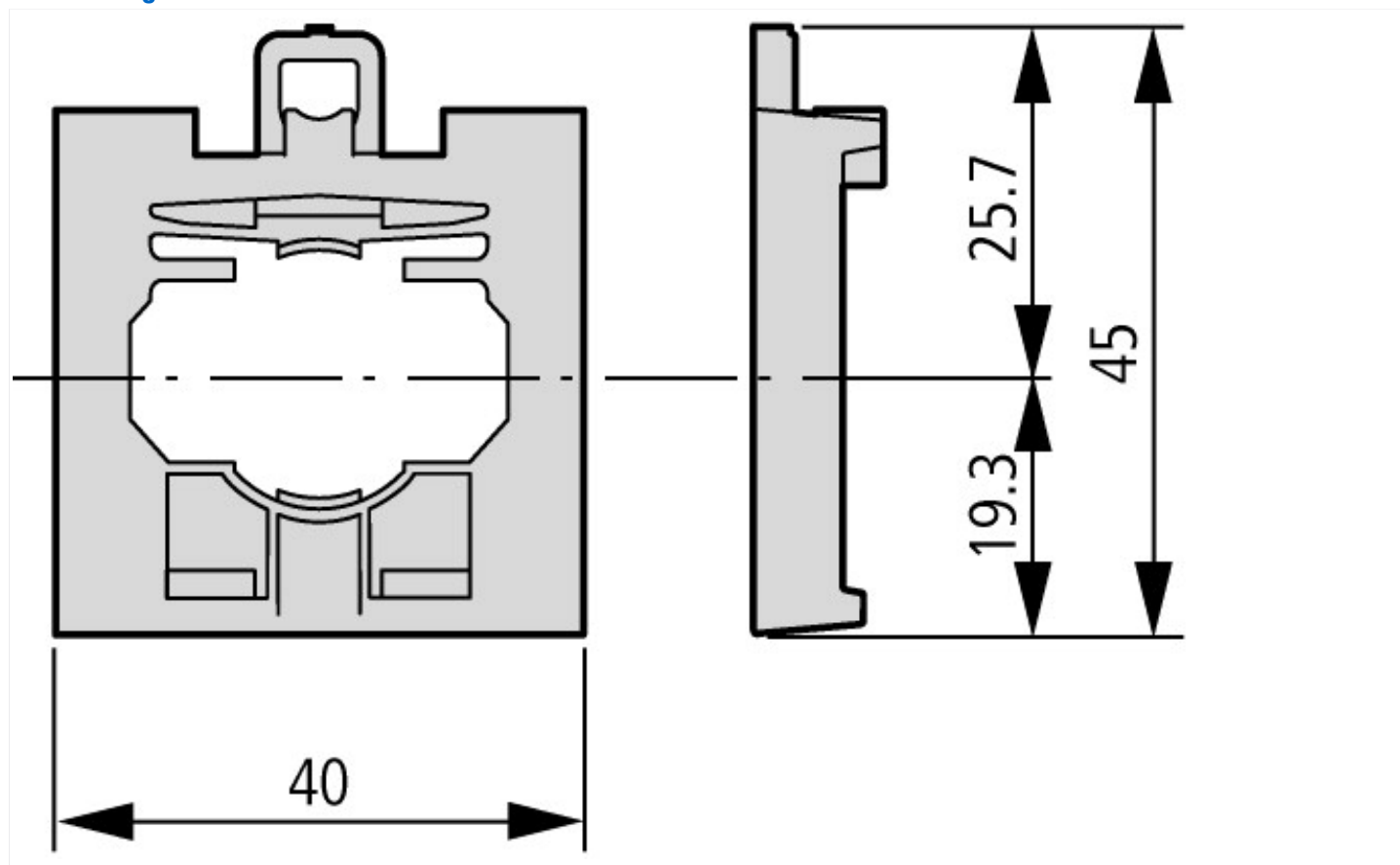
Befestigungsadapter Befestigungsadapter (Frontbefestigung) für 3 Kontakte-/LED-Elemente
