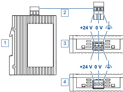
Abb. 3: 1) Geräteansicht (linke Seite), 2) Klemmblockansicht, 3) Geräteansicht (Oberseite): Anschluss am Gerät, 4) Geräteansicht (Oberseite): 3poliger Klemmblock gesteckt am Gerät
