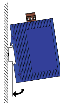
Abb. 5: Montage des SPIDER
