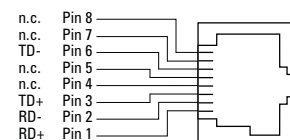
Abb. 2: Pinbelegung einer TP-Schnittstelle
