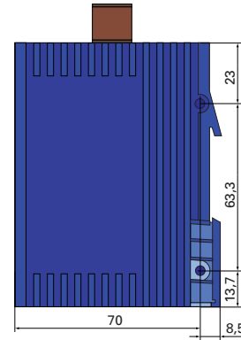
Abb. 6: Maße
