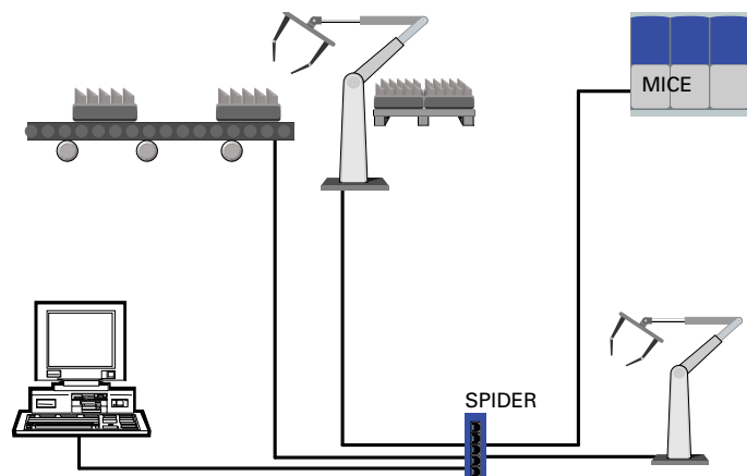
Abb. 4: Konfiguration mit SPIDER: Anschluss von – bis zu 8 Endgeräten oder weiteren Segmenten über TP (je nach Gerätevariante) u. – bis zu 1 Endgerät oder weiterem Segment über LWL (je nach Gerätevariante)
