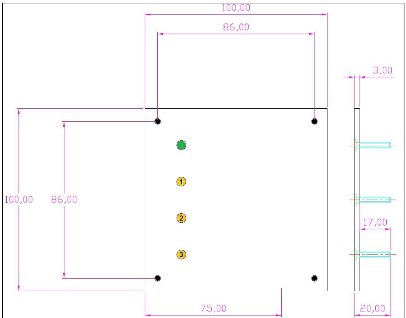
Abbildung 2: Maßbild
