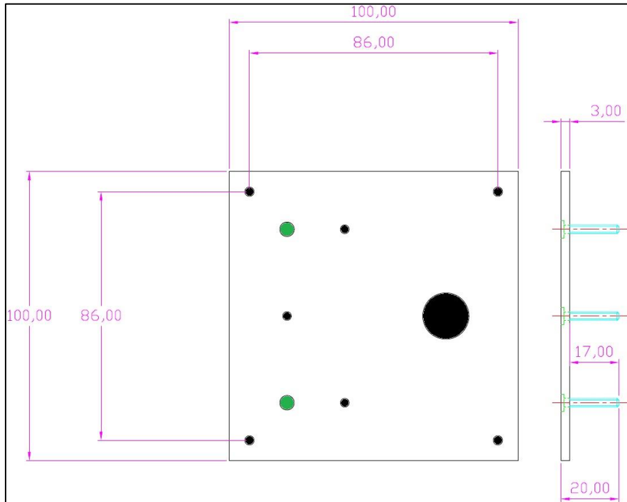
Abbildung 2: Maßbild
