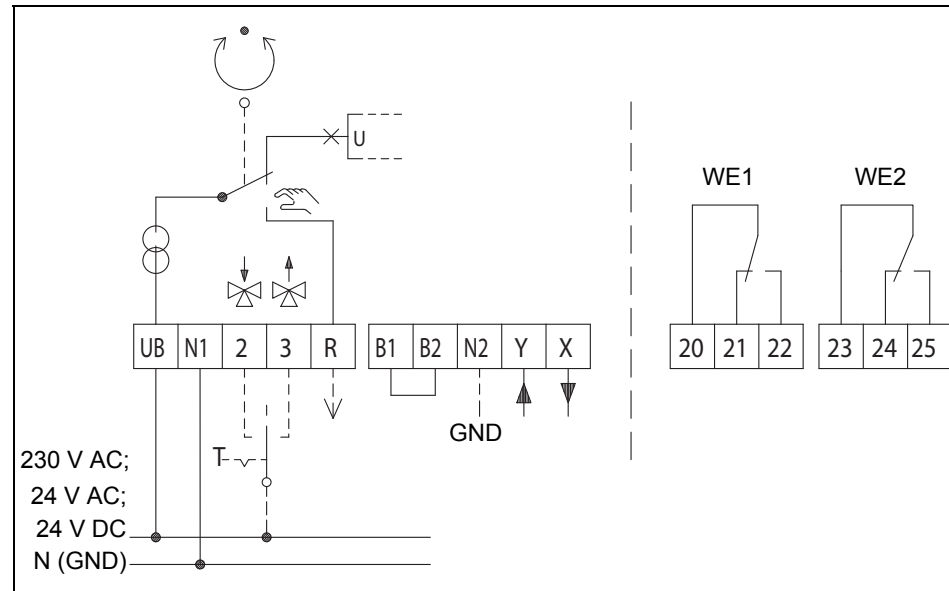
Bild 8 Schaltplan
