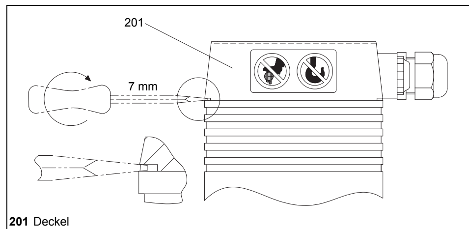
Bild 7 Deckel abnehmen
