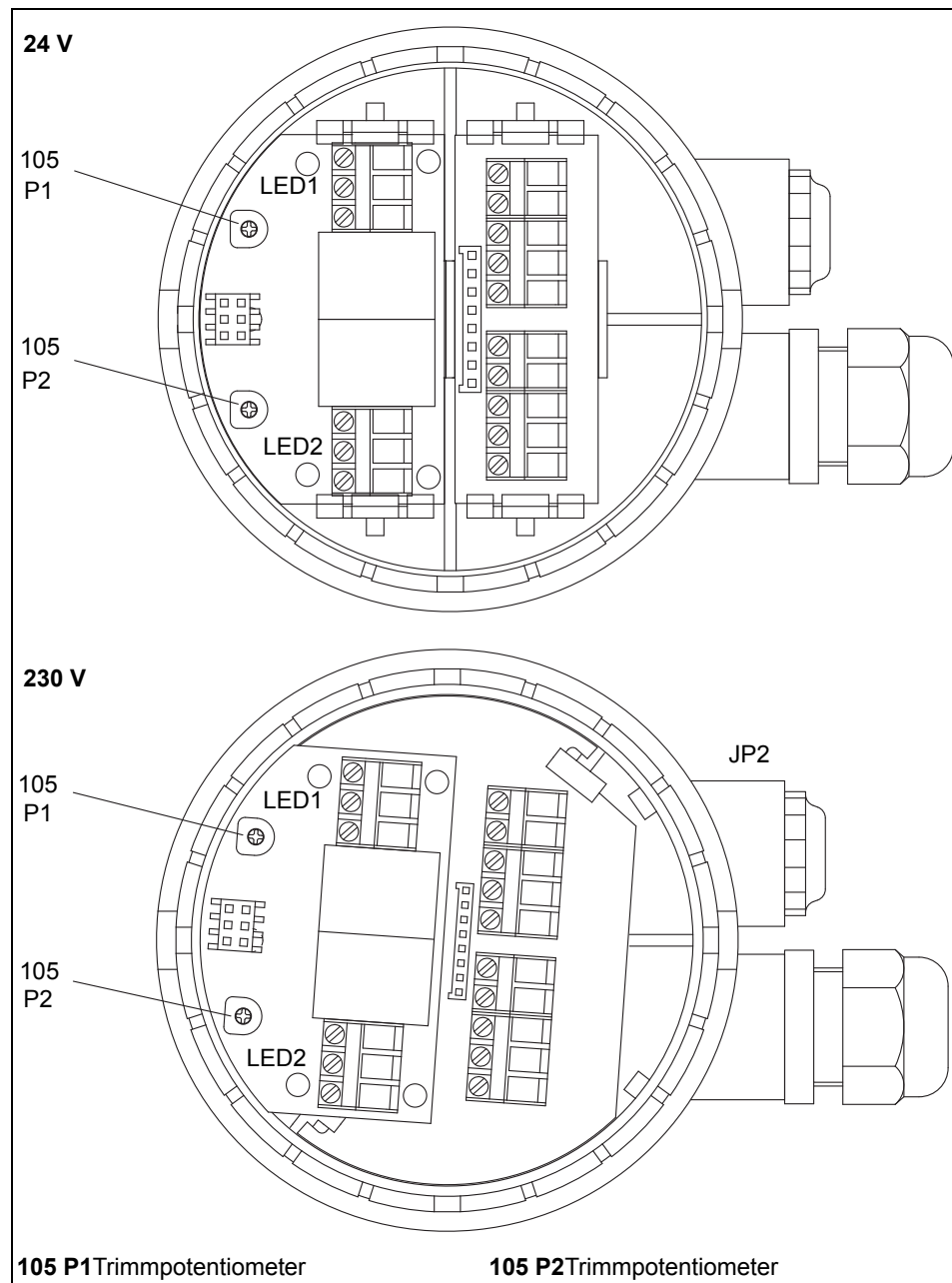
Bild 20 Wegschalterplatine im Deckel
