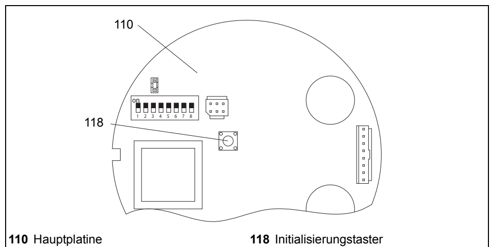
Bild 21 Wegmesssystem initialisieren
