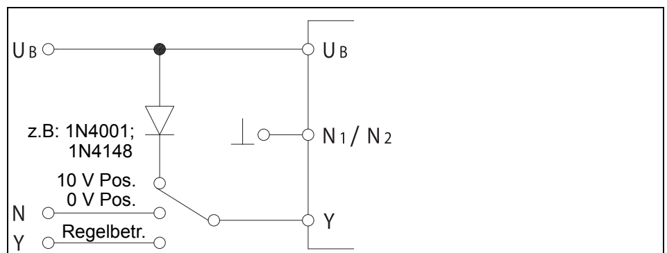
Bild 9 Reglerunabhängige Schaltung
