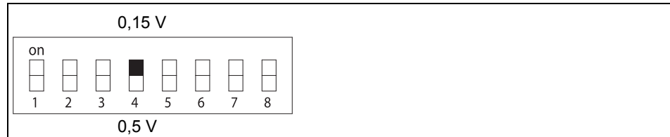
Bild 19 Hysterese einstellen
