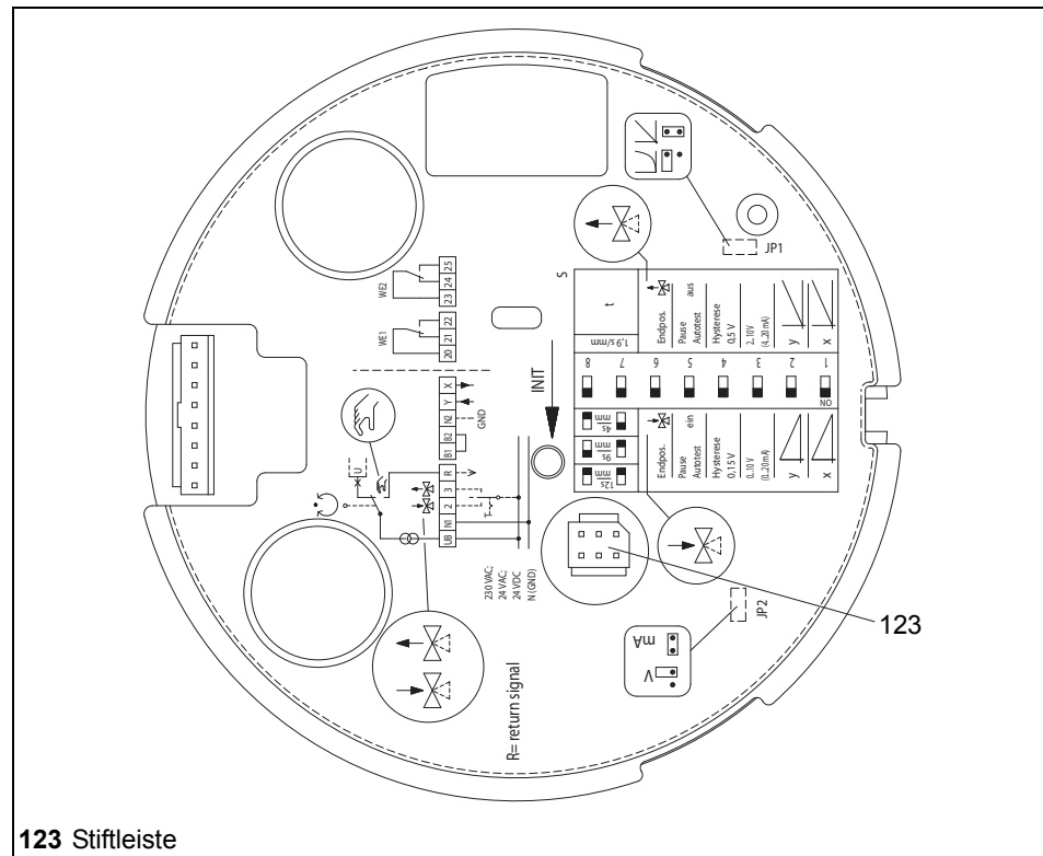
Bild 12 Stiftleiste für Weggshalterplatte auf der Hauptplatte
