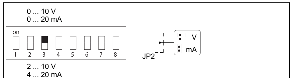
Bild 17 Eingangssignal einstellen
