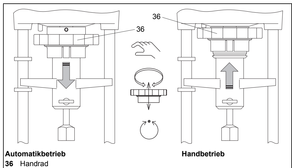
Bild 22 Automatikbetrieb wählen
