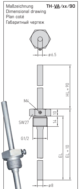
TH-VA/xx/90 Edelstahltauchhülse mit Halsrohr Stainless steel immersion sleeve with neck tube doigt de gant en acier inox avec tube prolongateur Гильза погружная из высококачественной стали с горловиной
