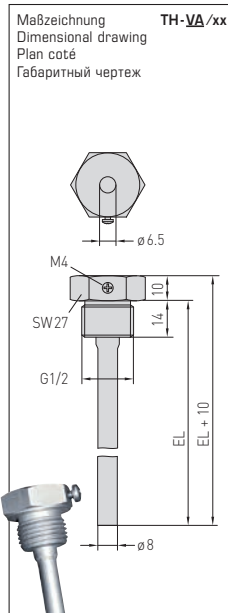
TH-VA/xx Edelstahltauchhülse Stainless steel immersion sleeve doigt de gant en acier inox Гильза погружная из высококачественной стали
